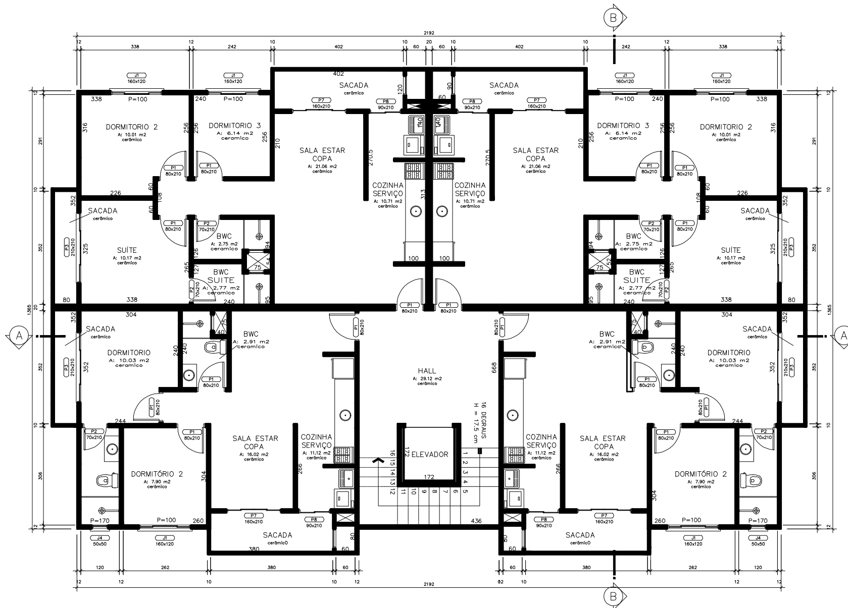
PLANTA BAIXA PVTO TIPO 4X Escala 1/50
